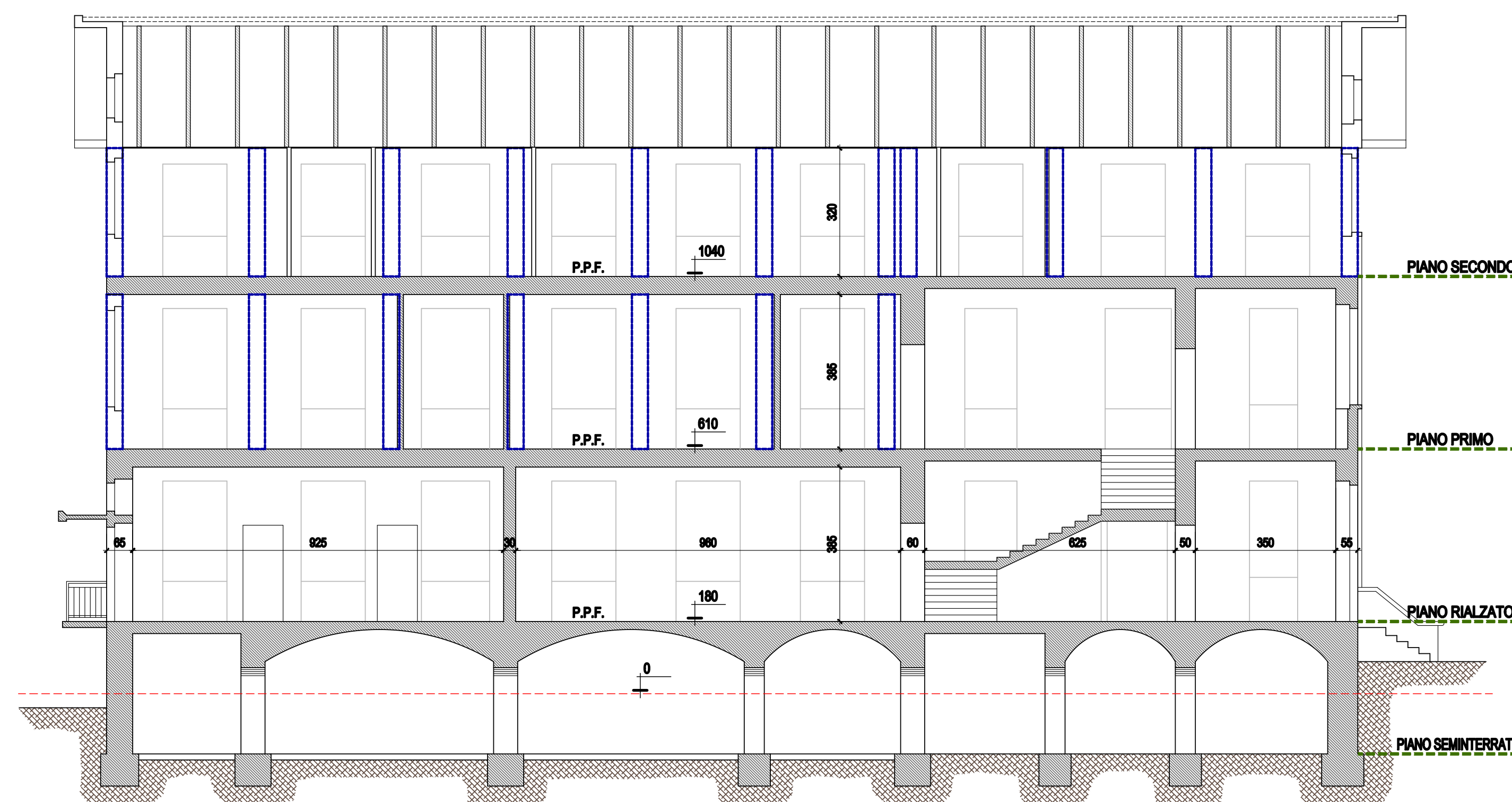
SEZIONE C-C
