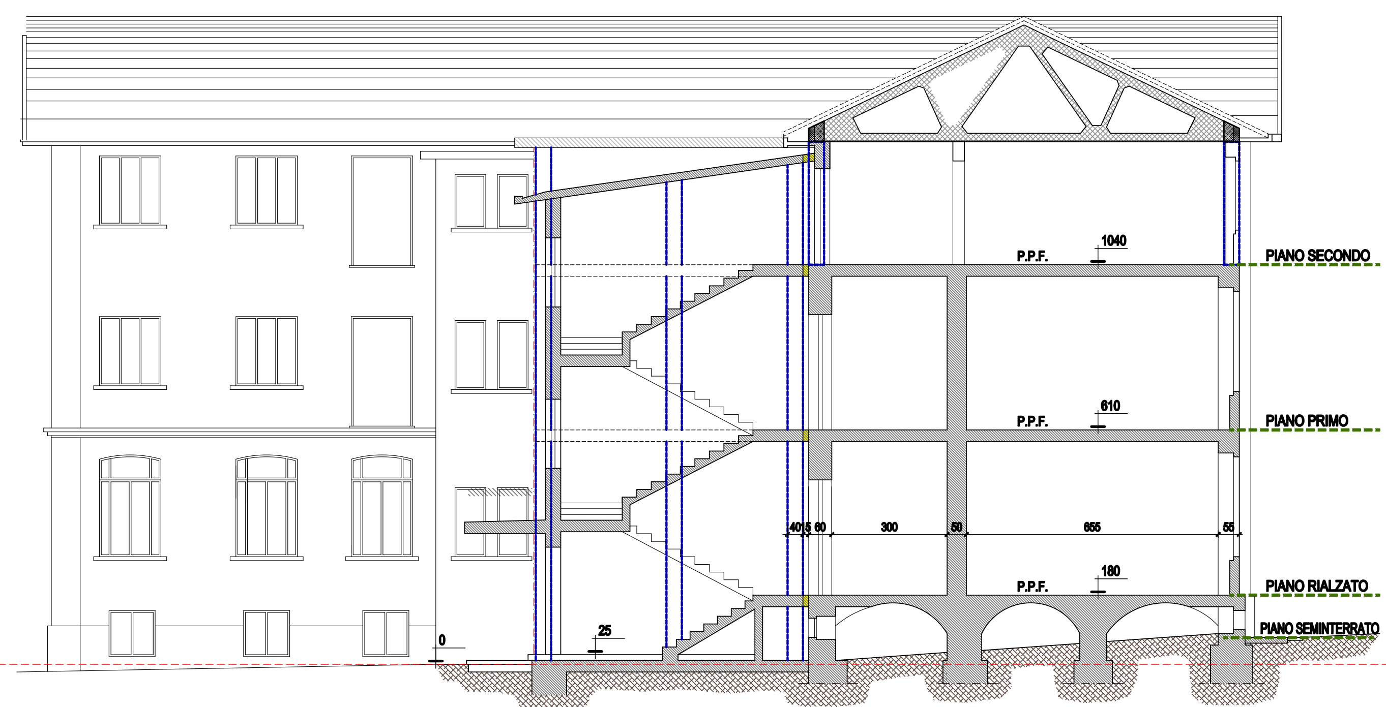
SEZIONE B-B
