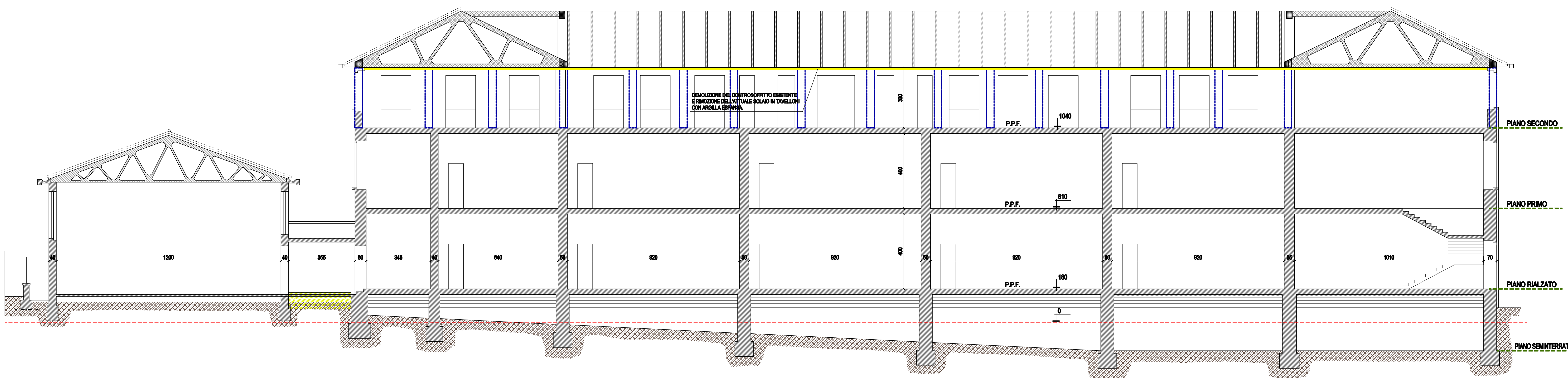
SEZIONE A-A
