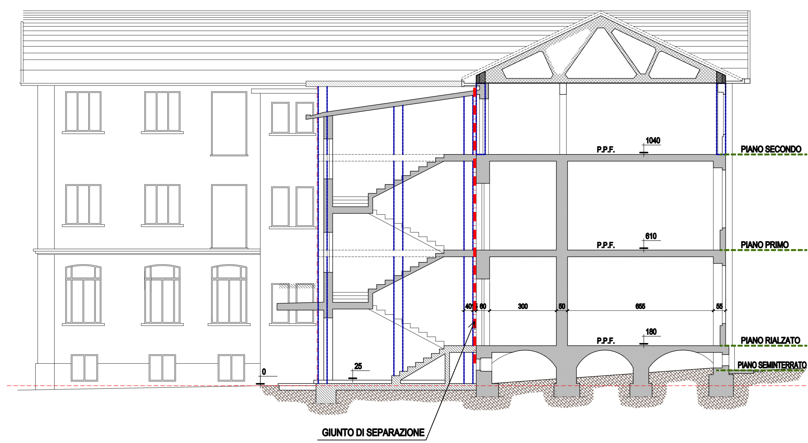
SEZIONE B-B
