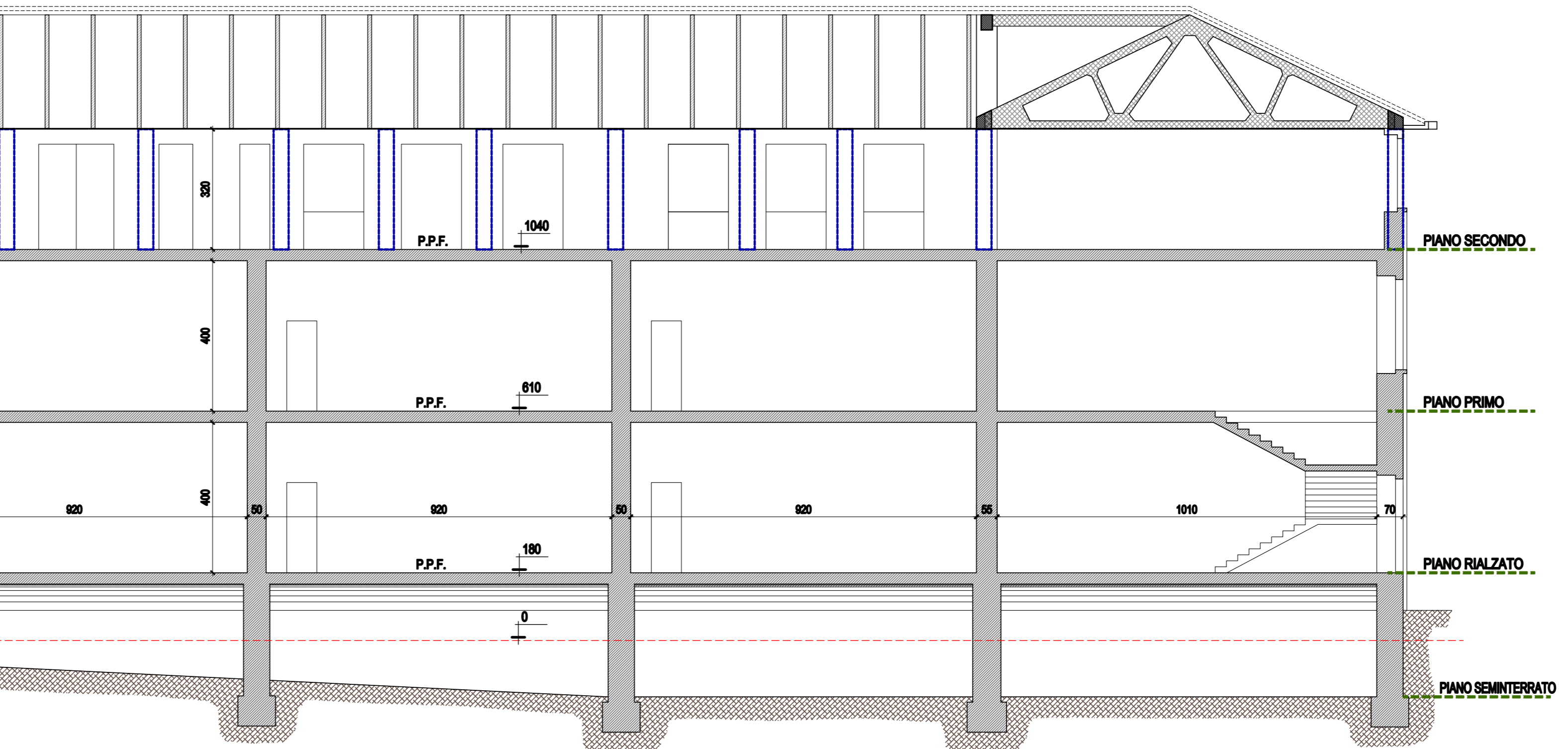
SEZIONE C-C
