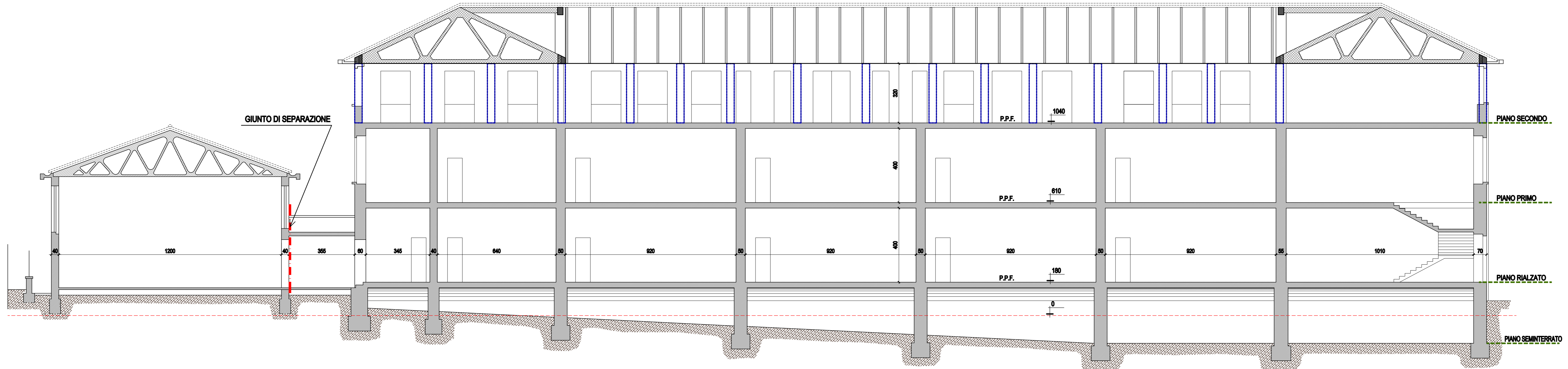
SEZIONE B-B
