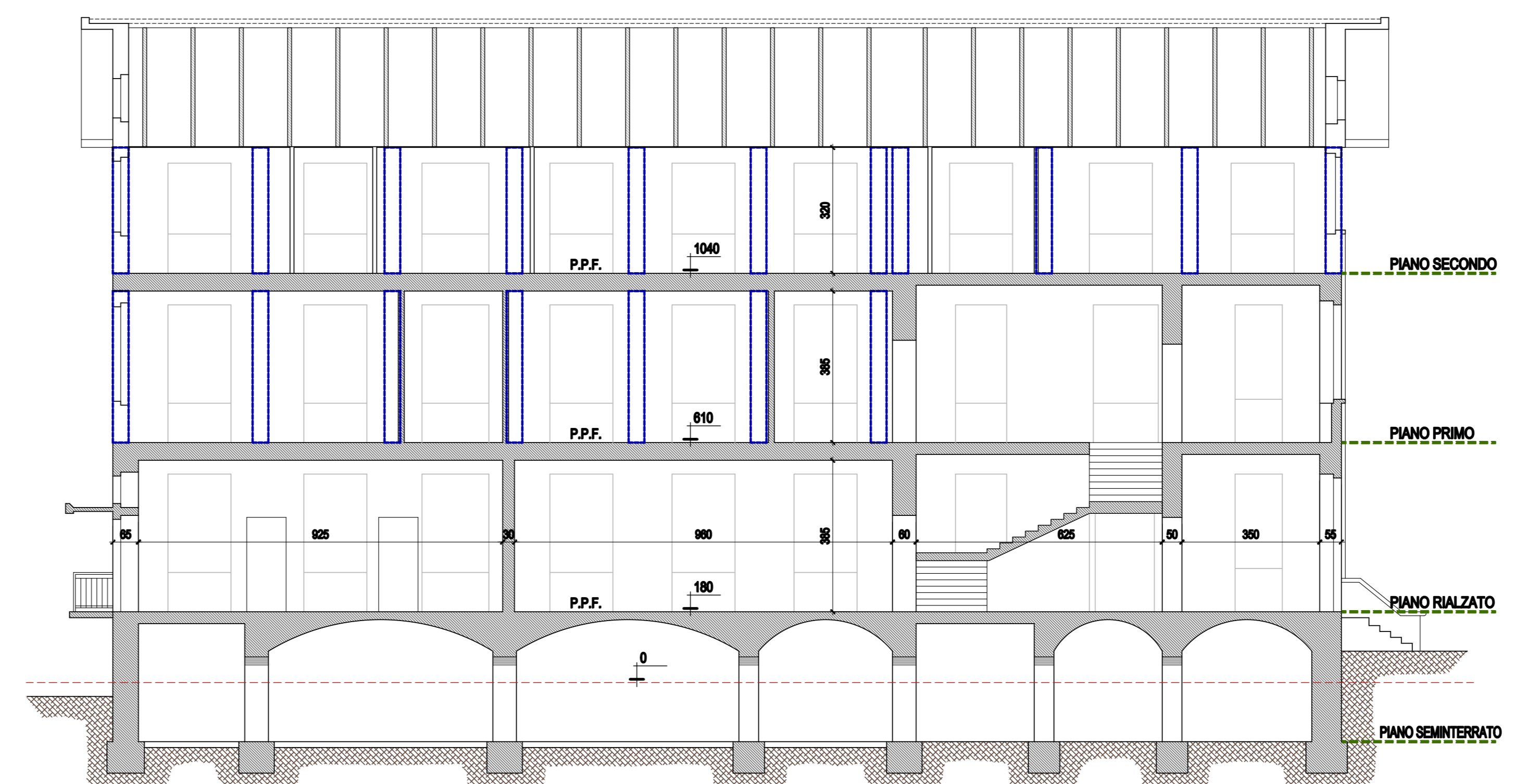
SEZIONE C-C
